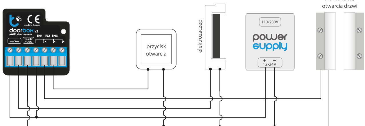
2. Schemat podłączenia kontaktronu - magnetycznego czujnika otwarcia drzwi
